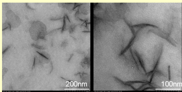
Cu whisker particles 50~100nm
